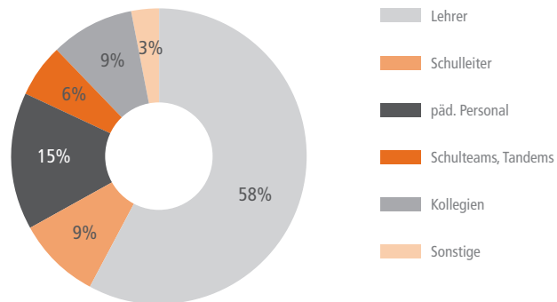
Abbildung 3: Trend: Adressaten
